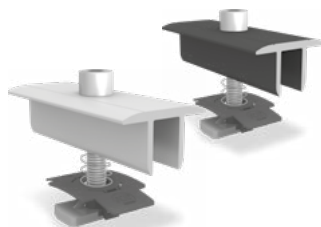
XS Étrier intermédiaire aluminium/noir anodisé
