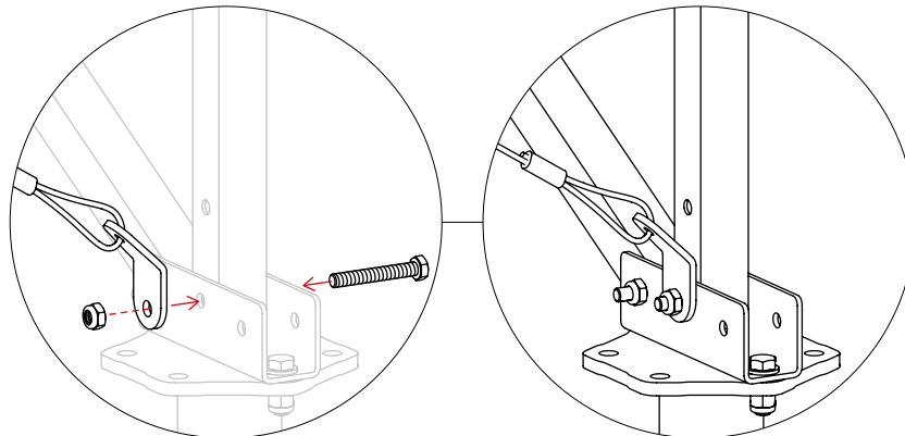
Fondations vissées
