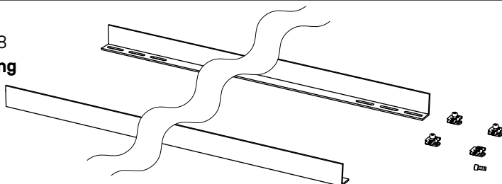
1001643 + 2001729 Tassello scorrevole MK2 con clip + Vite a testa cava esagonale M8×20
