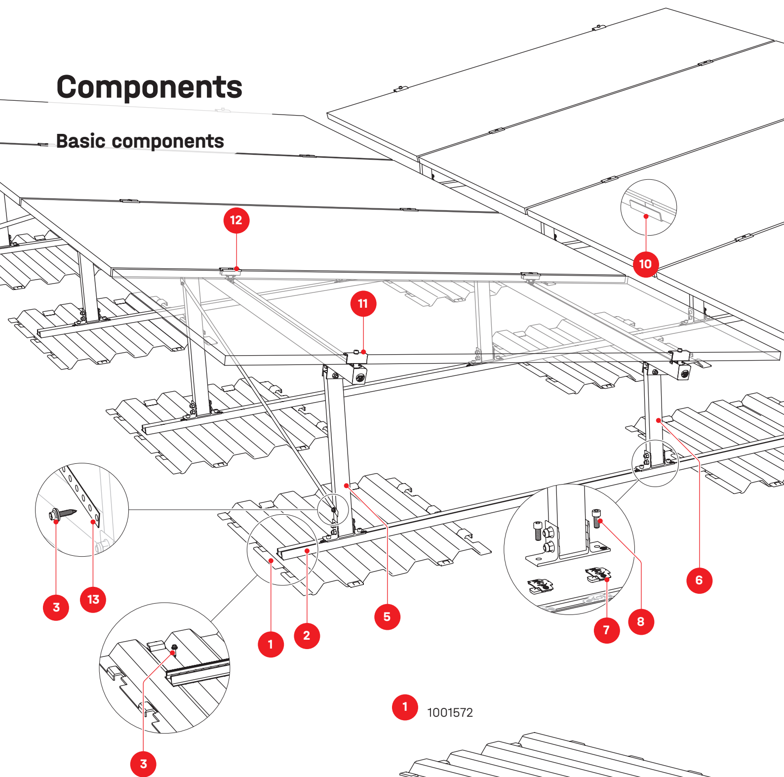
PE Baseplate
